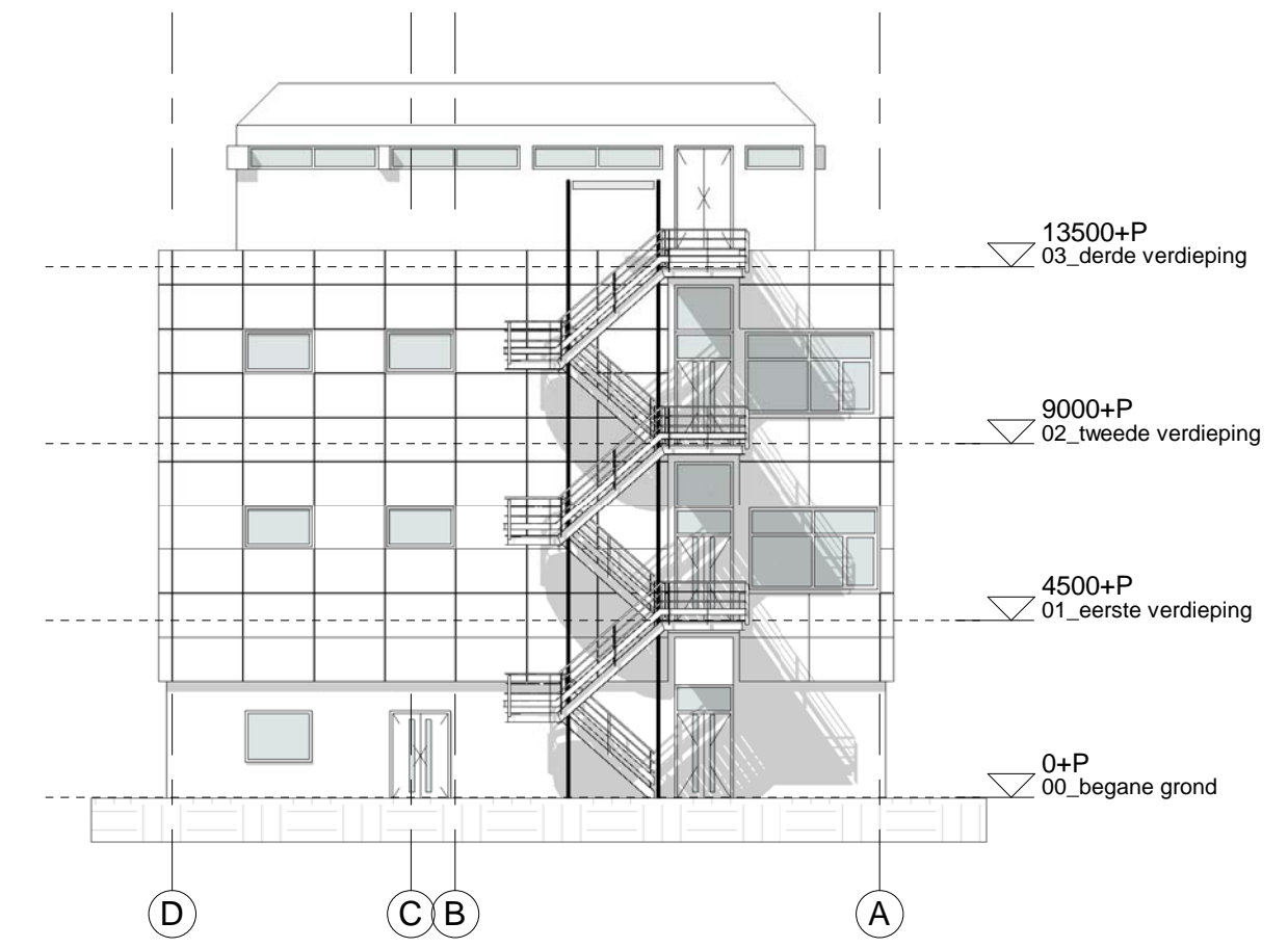
308_gevelaanzicht zuid bestaand
