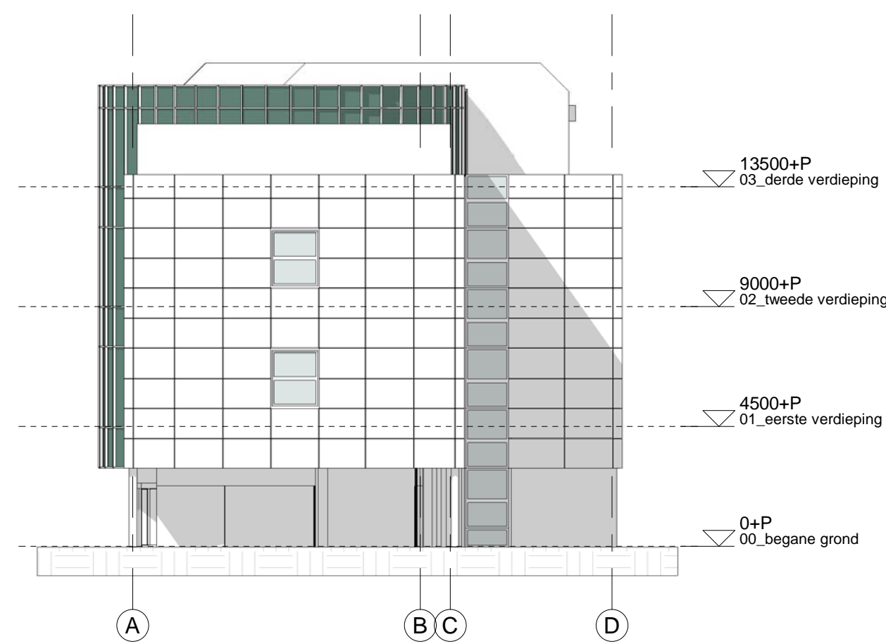
306_gevelaanzicht noord bestaand
